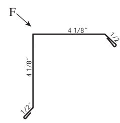
Ⓓ 29 Ga. AG4 Gable Trim 10'2" TLFS17xx
