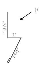
Ⓔ 29 Ga. Base Angle 10'2" TLBA3xx
