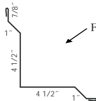
Ⓜ 29 Ga. Inside Corner 10'2" TLIC13xx
